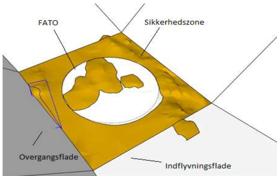
Billede 1: Hindringer ved helikopterflyveplads og ved ind- og udflyvningsflade
