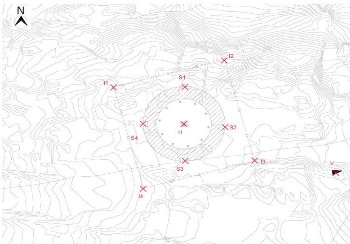
Billede 1: Hindringer ved helikopterflyveplads og ved ind- og udflyvningsflade
